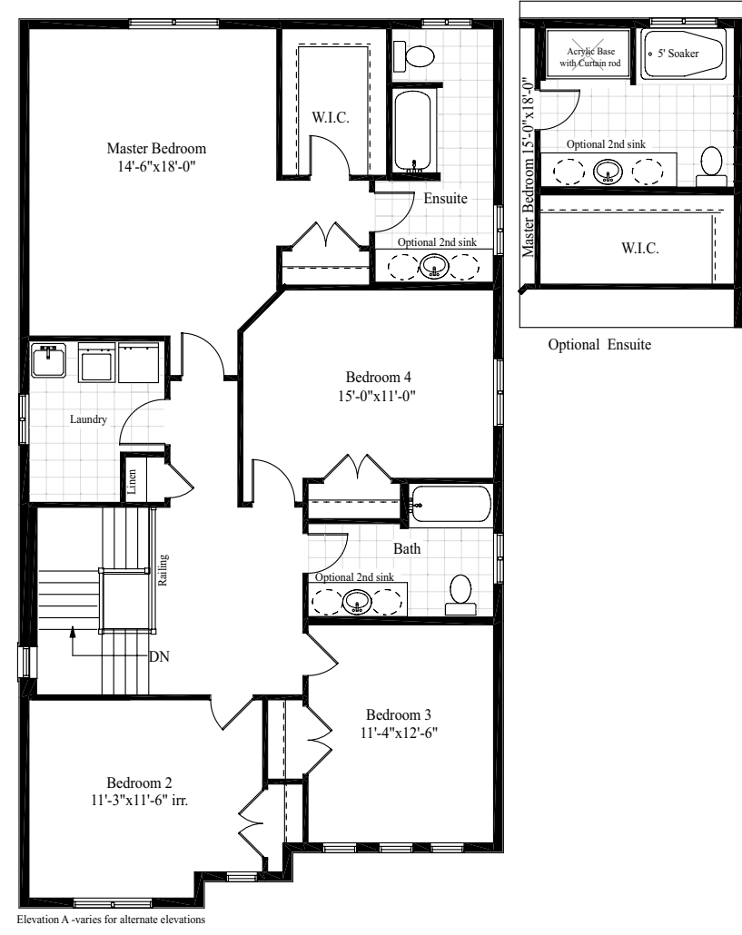
Elevation A
